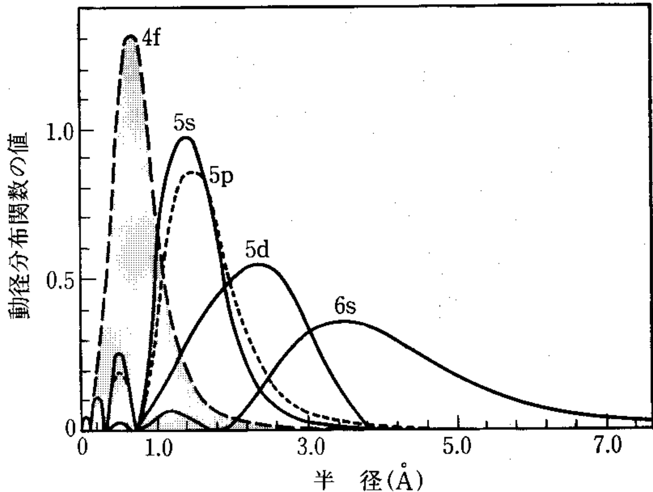
図1.1 4f, 5s, 5p および 6s 軌道の空間的な広がり
